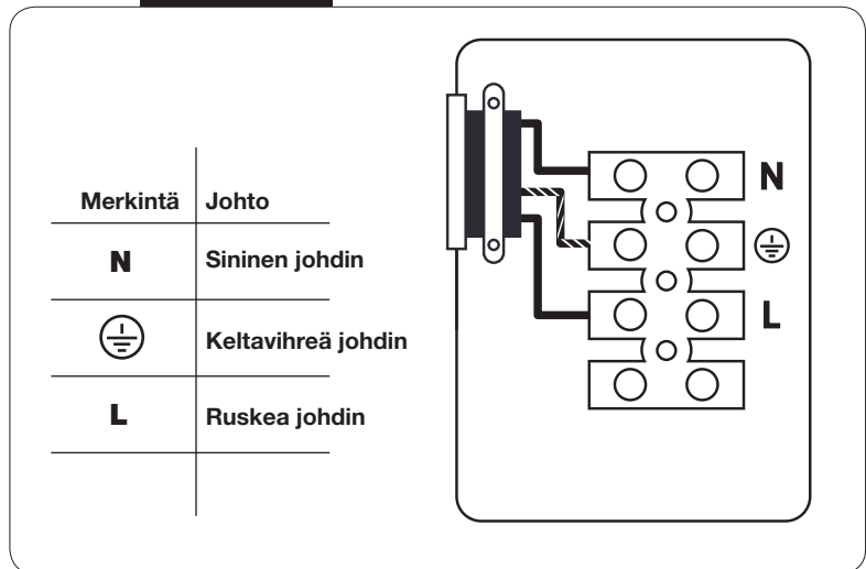
Fig: 2 Sähköliitännät
